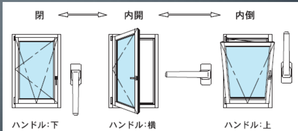
ドレーキップ
