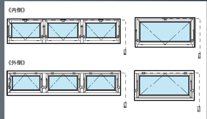
外倒し・内倒し (ホーラー可)
