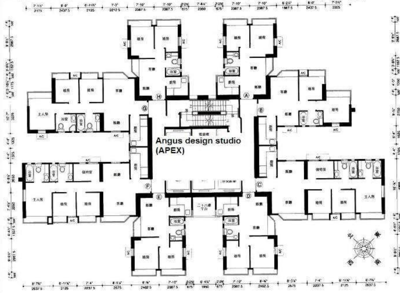
Block 1 5th-48th Floor Plan 第1座 五至四十八樓平面圖
