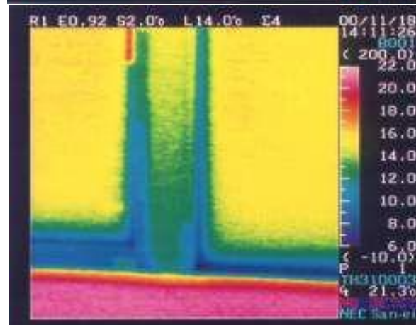
アルミ熱遮断構造
