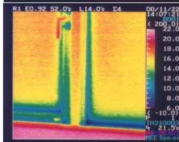
アルミ樹脂複合
